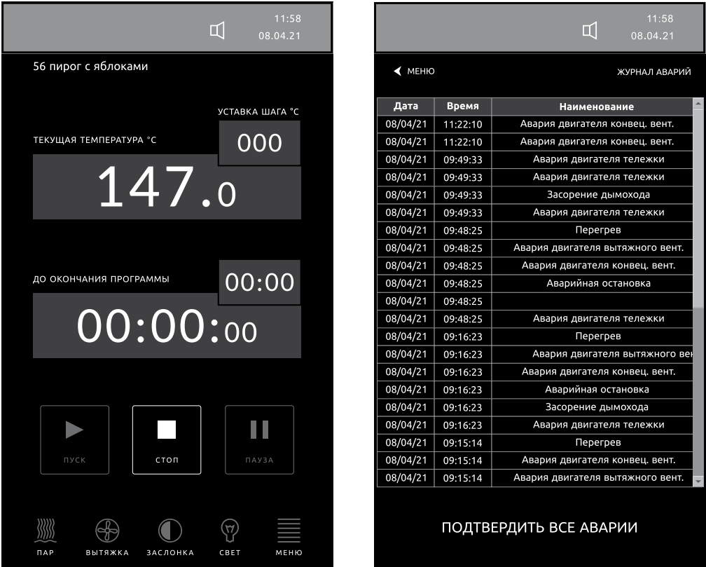
Рисунок 37 - Режим аварийной ситуации
