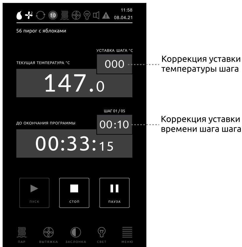
Рисунок 5 - Коррекция уставок температуры и времени
